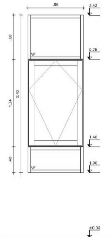
Ejemplo de abertura tipo "A10"
